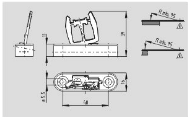
Desenho dimensional (geral)
