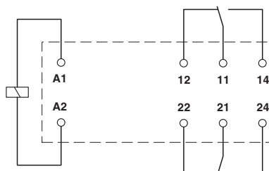
Diagrama de circuitos
