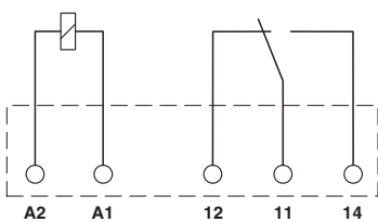
Diagrama de circuitos
