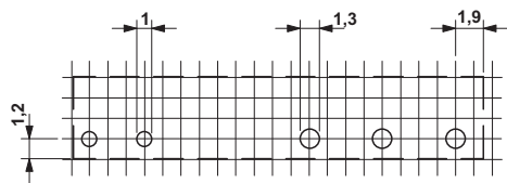
Esquema de perfuração
