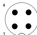
Desenho dos contatos conector M12, 4 pólos, codificação A, vista lado do pino
