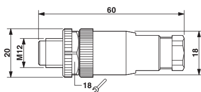
Conector M12 x 1, reto
