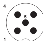
Conector Polbild M12, 5 pólos, codificação A, vista lado do suporte
