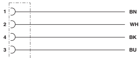
Diagrama de circuitos
